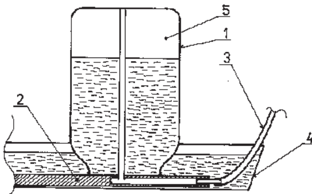
Obr. č. 7 Schéma vodního plynojemu pro jímání bioplynu (1 sekce)
